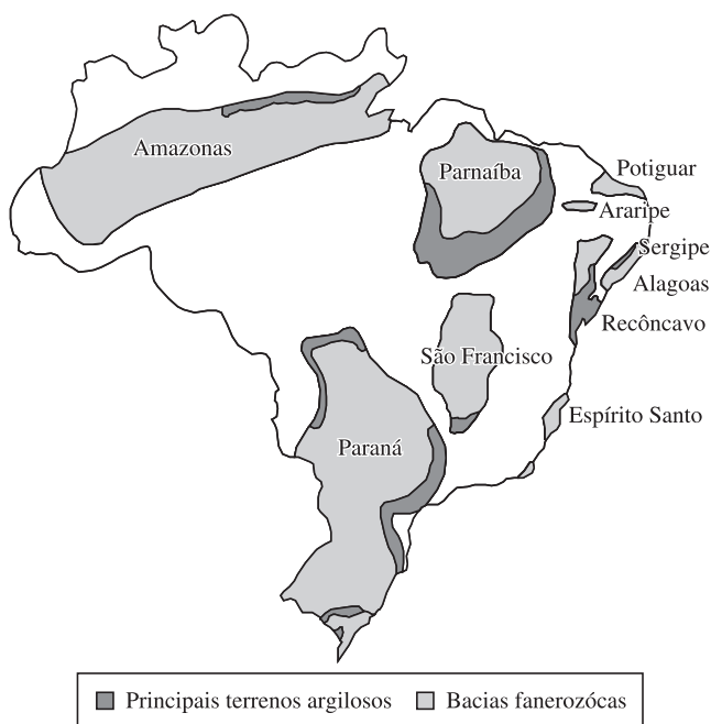
Figura 3. Distribuição das principais bacias sedimentares brasileiras portadoras de depósitos de argila para uso em cerâmica vermelha. Fonte: modificado de Motta 13 .
