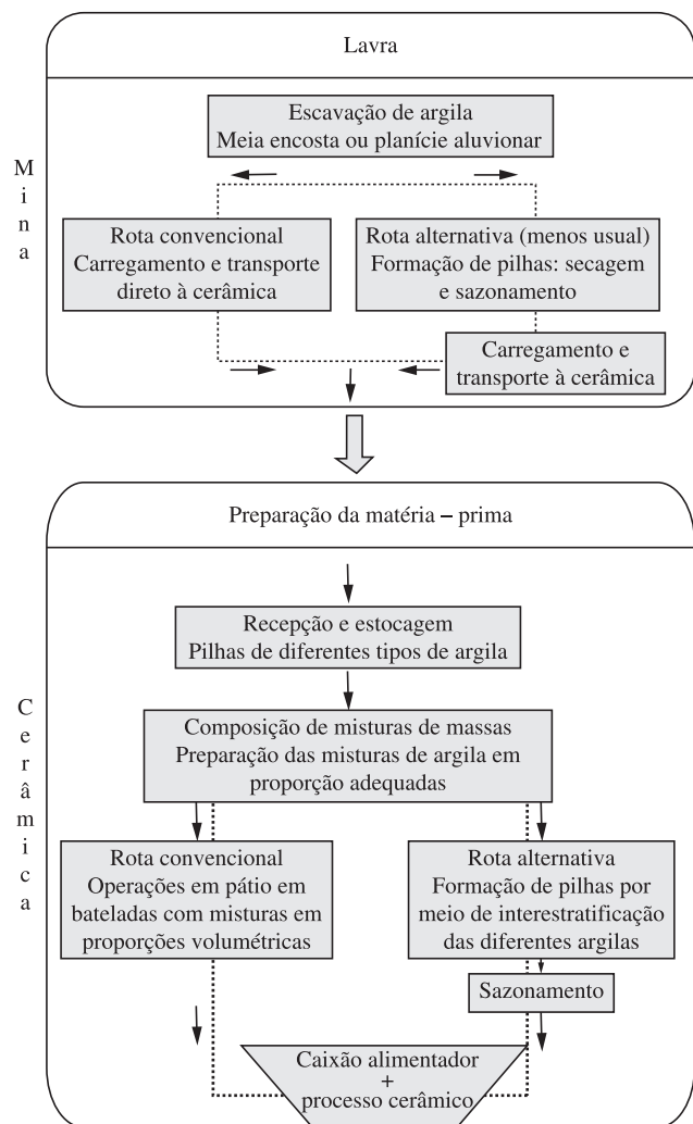
Figura 5. Fluxograma das operações unitárias da produção de argila e preparação de massa cerâmica.
